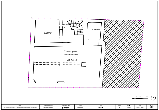
Sous-sol
