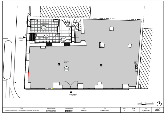
RDC
